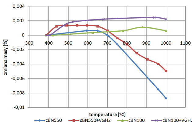
Rys. 3. Nieizotermiczne zmiany masy ziaren ściernych z cBN
