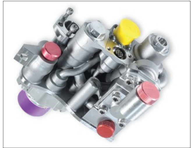
Fig. 4. 3D printed titanium alloy valve block (source: Liebherr) Rys. 4. Wydrukowany w technologii druku 3D ze stopu tytanu blok zaworowy (źródło: Liebherr)
