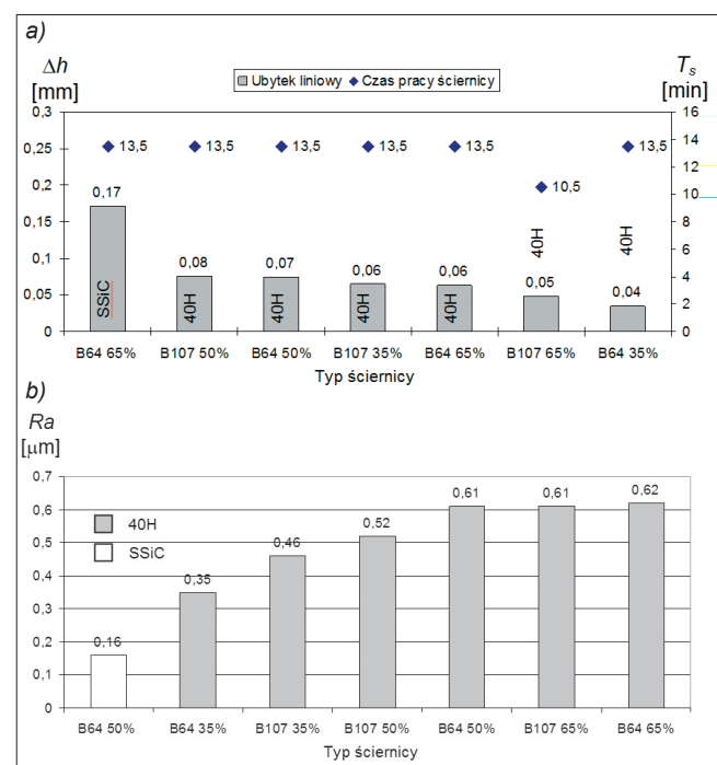
Rys. 1. Efekty technologiczne szlifowania jednostronnego: a) całkowity liniowy ubytek materiału obrabianego oraz czas pracy ściernic z ziarnami z regularnego azotku boru – uszeregowanie ściernic według malejącego ubytku \Delta h , b) wartość końcowa parametru chropowatości R_a – uszeregowanie ściernic według rosnącej wartości parametru R_a
