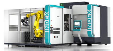
Centrum tokarsko-frezarskie INDEX G420 z robotem iXcenter do wydajnej obróbki dużych detali
