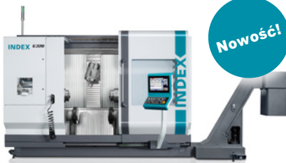
Centrum tokarsko-frezarskie INDEX G220 do elastycznej i wysoko wydajnej obróbki
